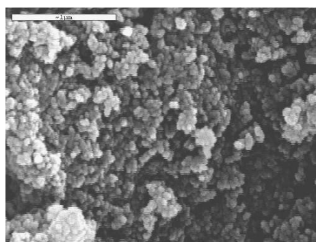
图 2 纳米球型碳酸钙 (50~60 纳米)
