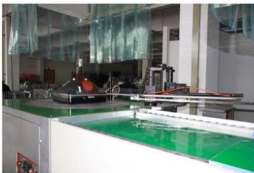
上图 自主研发了自动缠绕电加热 CRT 锥屏分离方法及设备 (可实现高效无损分离, 分离效率为 2 分钟/台)
