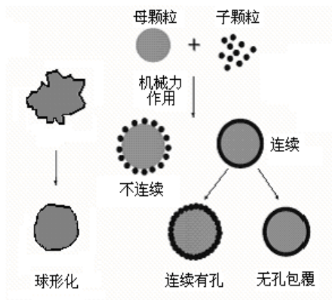
上图 生产功能性微纳米复合粉体材料的技术路线
