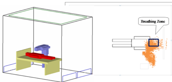
图3 医疗环境中传染病控制环境设计
